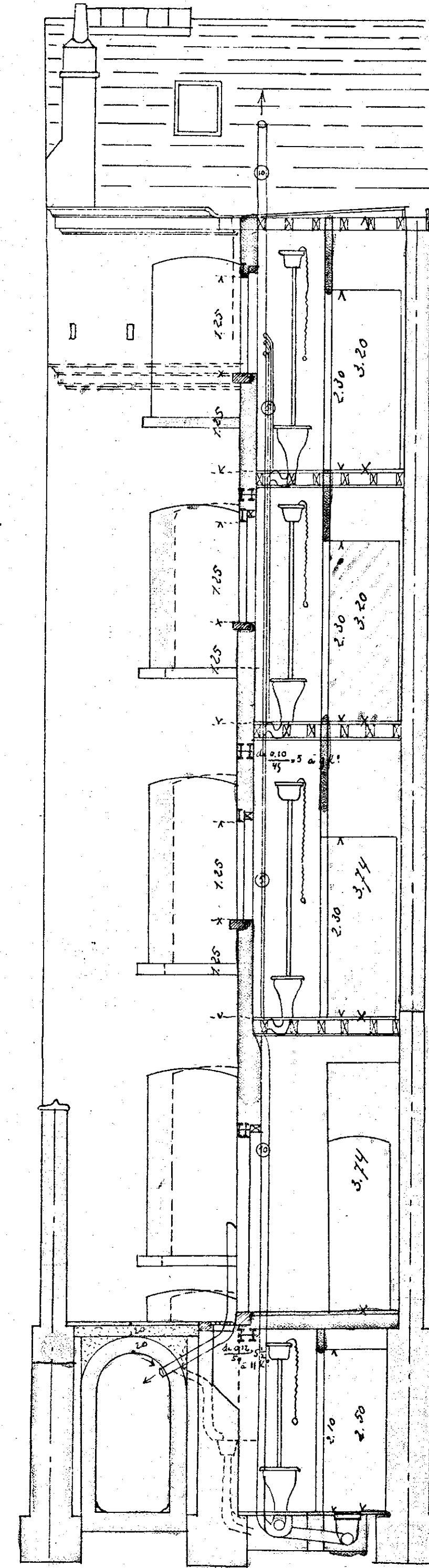
- Coupe A-B -
